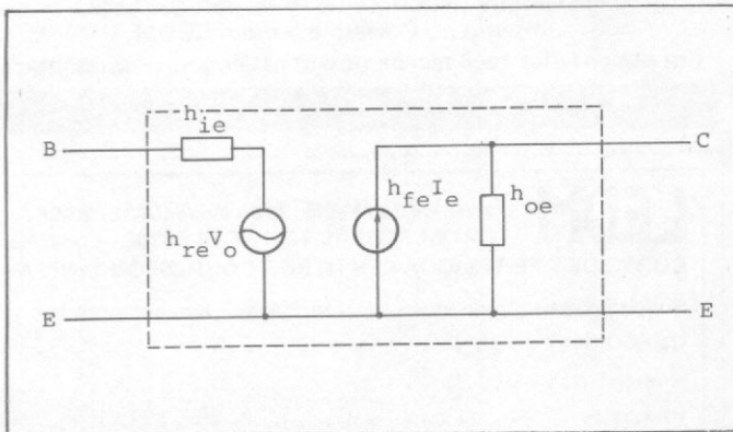
Figura 2 - Equivalente híbrido do transistor
